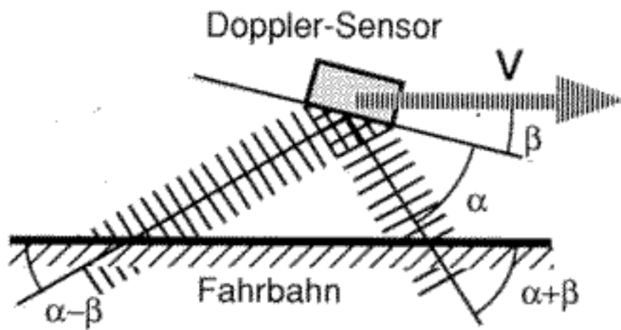
Bild 2: Kompensation von Verkippungen ( \beta ) des Sensors durch eine sog. "Janus"-Antenne
