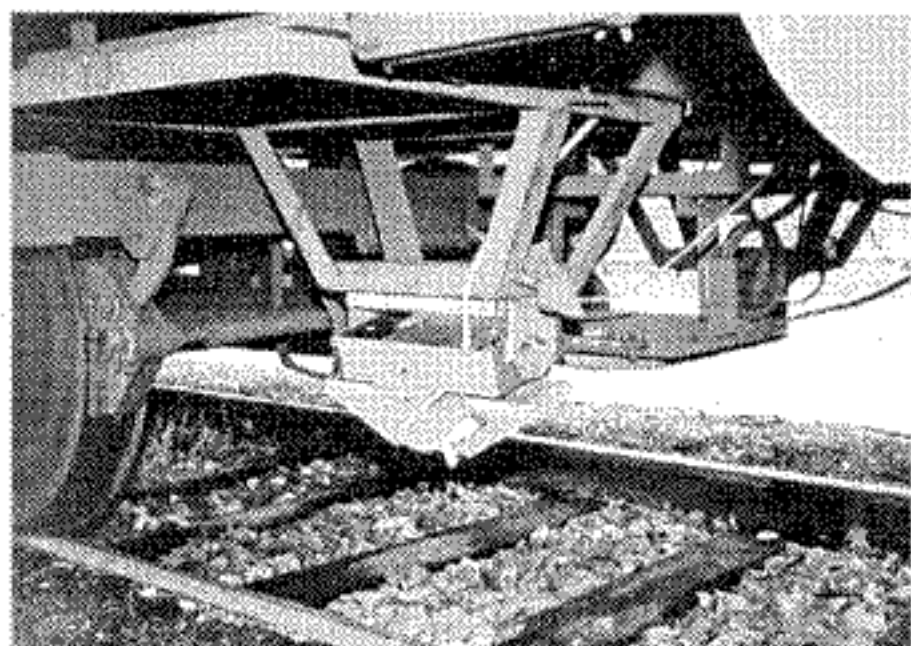
Bild 4: Doppler-Sensor im bahntauglichen Gehäuse an der Unterseite eines Eisenbahnwagens
