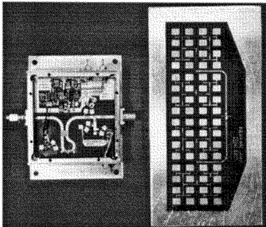
Bild 3: Dielektrisch stabilisierter 24 GHz-Grundwellenoszillator und "Janus"-Antenne [3].
