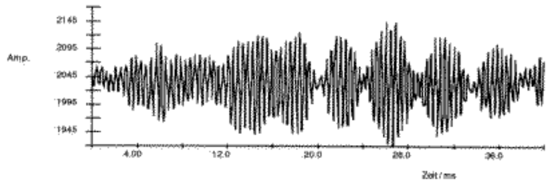
Bild 7: Doppler-Rohsignale in unterschiedlichen Zeitmaßstäben, ein Wellenzug entspricht einem Anteil von ca 9 mm der gesamten Zuglänge
