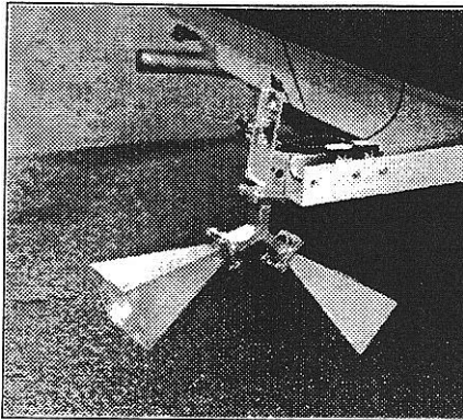
Bild 7: Am Kfz montierter 10 GHz-Janus-Mikrowellensensor
