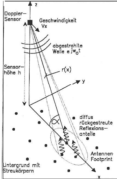
Bild 1: Berührungslose Messung der Geschwindigkeit über Grund mit Doppler-Sensor
