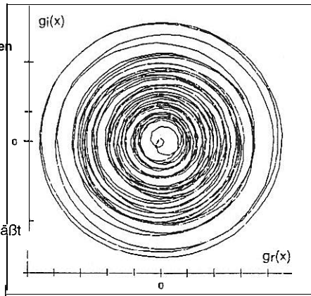
Bild 4: Verlauf des komplexen Dopplersignalzeigers g(x) bei Bewegung des Sensors
