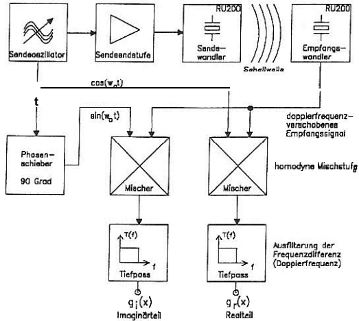
Bild 3: Blockschaubild des Ultraschall-Dopplersensors mit komplexem Ausgangssignal g(x) = g_r(x) + jg_i(x)
