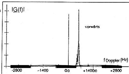
Bild 5: Dopplerspektrum |G(f)| für Bewegung vorwärts
