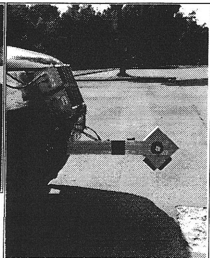
Bild 8: Am Kfz montierter 200 kHz-Janus-Ultraschallsensor
