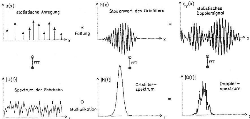
Bild 2: Systemtheoretische Darstellung des Dopplersensors als Ortsfrequenzfilter
