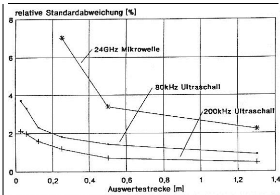
Bild 6: Relative Standardabweichung von 50 Geschwindigkeitsmeßwerten bezogen auf den Mittelwert (Nullstellenauswertung) in Abhängigkeit der Auswertestrecke. Vergleich des Meßfehlers für Ultraschall- und Mikrowellen-Dopplersensoren
